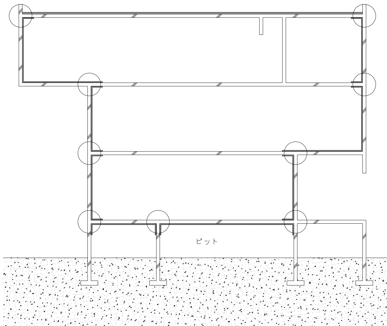
(a)屋根-外断熱、外壁-内断熱の構造熱橋部
