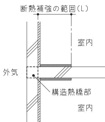
(b)構造熱橋部
