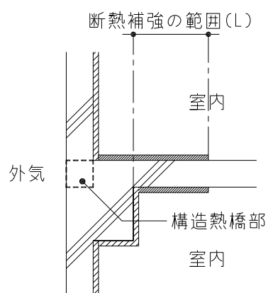
(c)構造熱橋部 内梁
